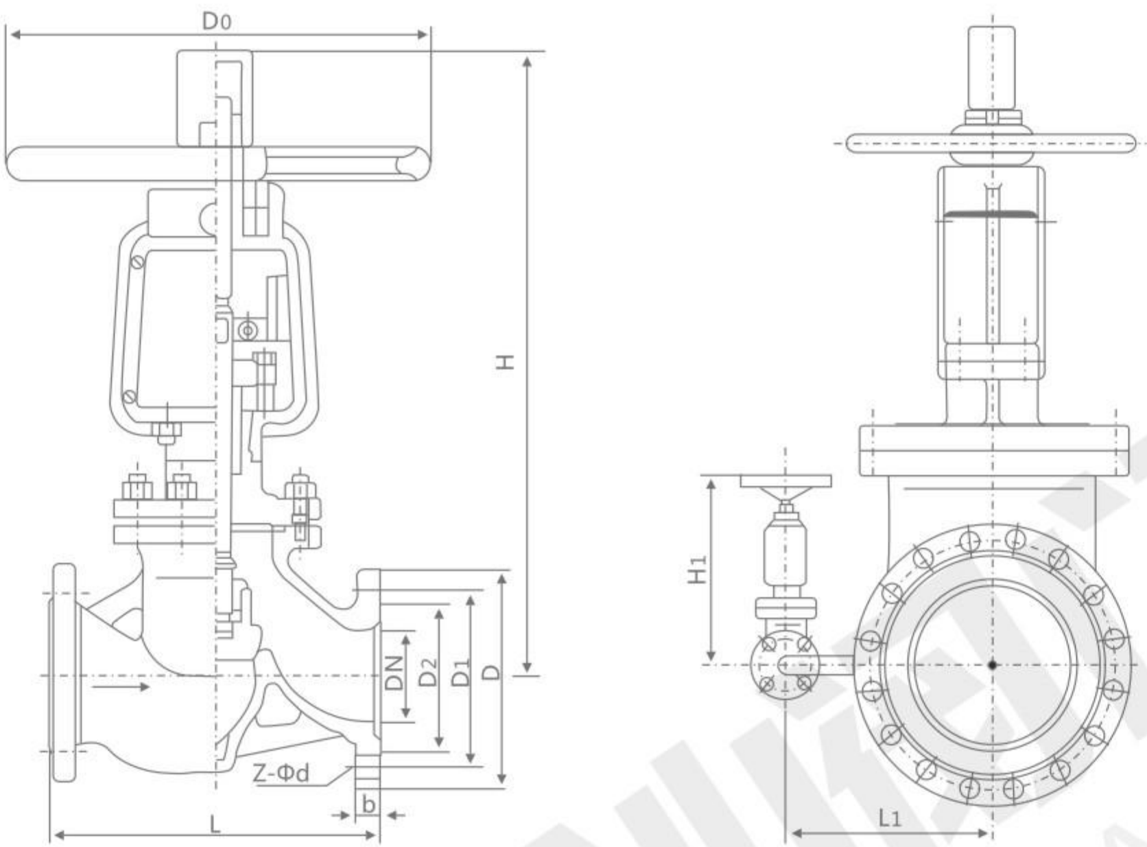
主要外形及和连接尺寸 Main external and connection dimension JB/T79.1 单位Unit:mm
