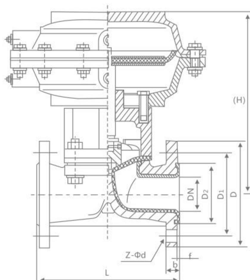
Eg641 F 46 型气动隔膜阀(堰式)
