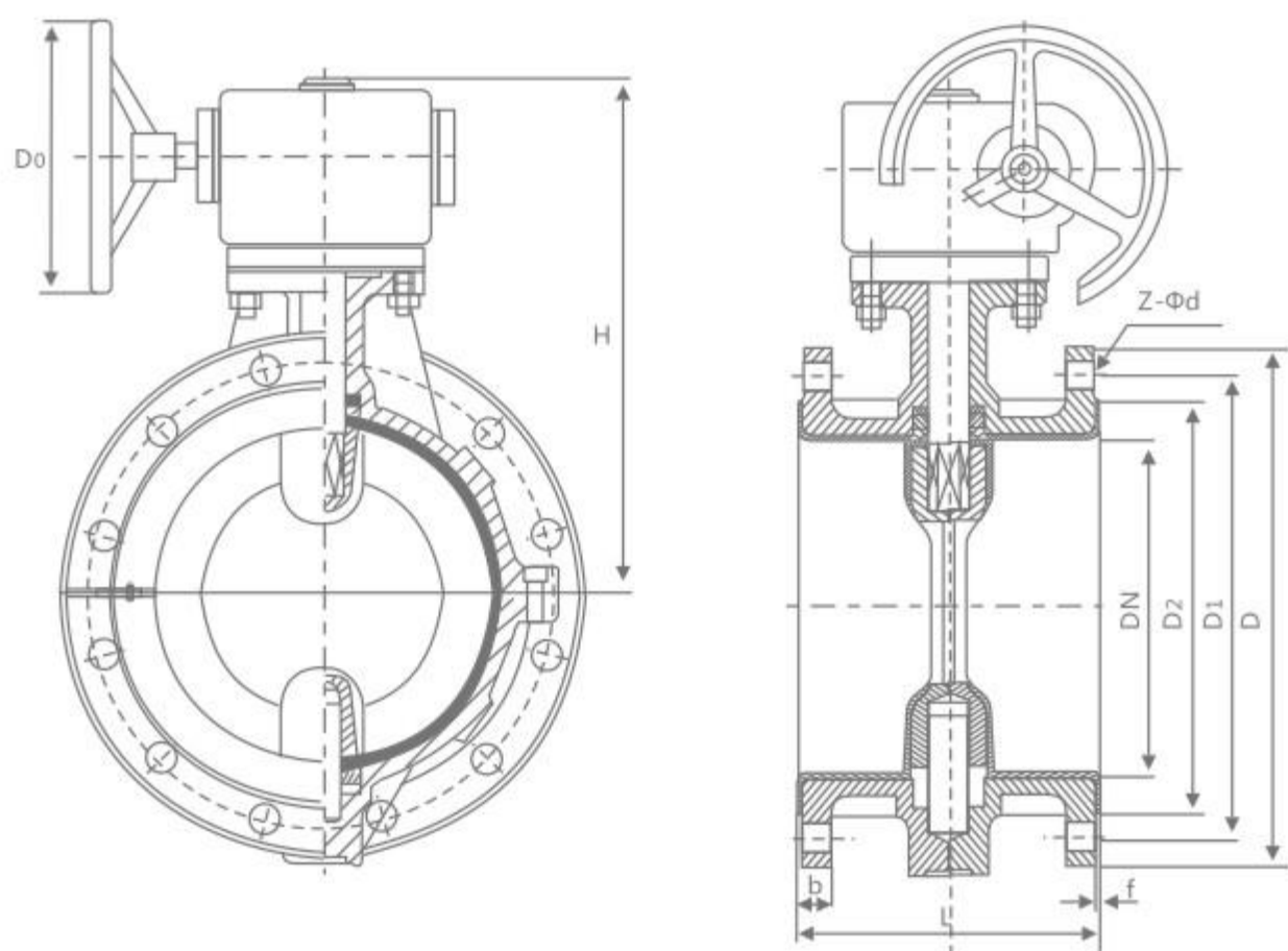
DA341F 46 型法兰连接蜗轮传动蝶阀 (中线)
